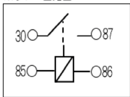
※リレー回路図
