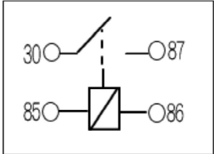
※リレー回路図
